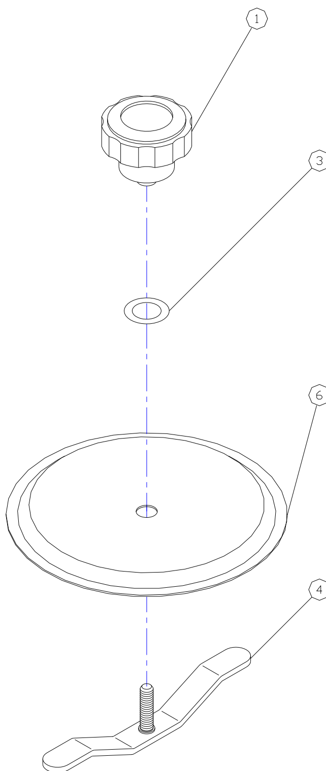
LID ASSEMBLY (PART # 500320)
