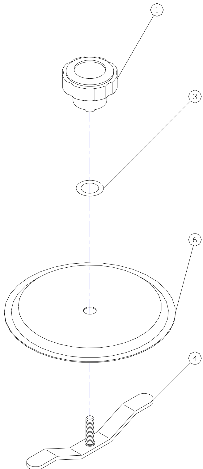
LID ASSEMBLY (PART # 500320)
